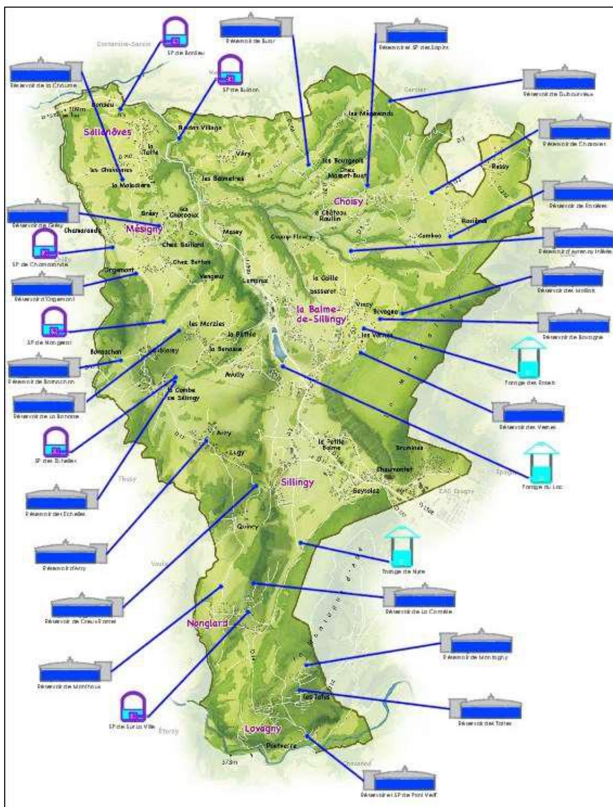
Positionnement des ouvrages de stockage et de pompage de la CCFU (capture issue du logiciel de télégestion)
